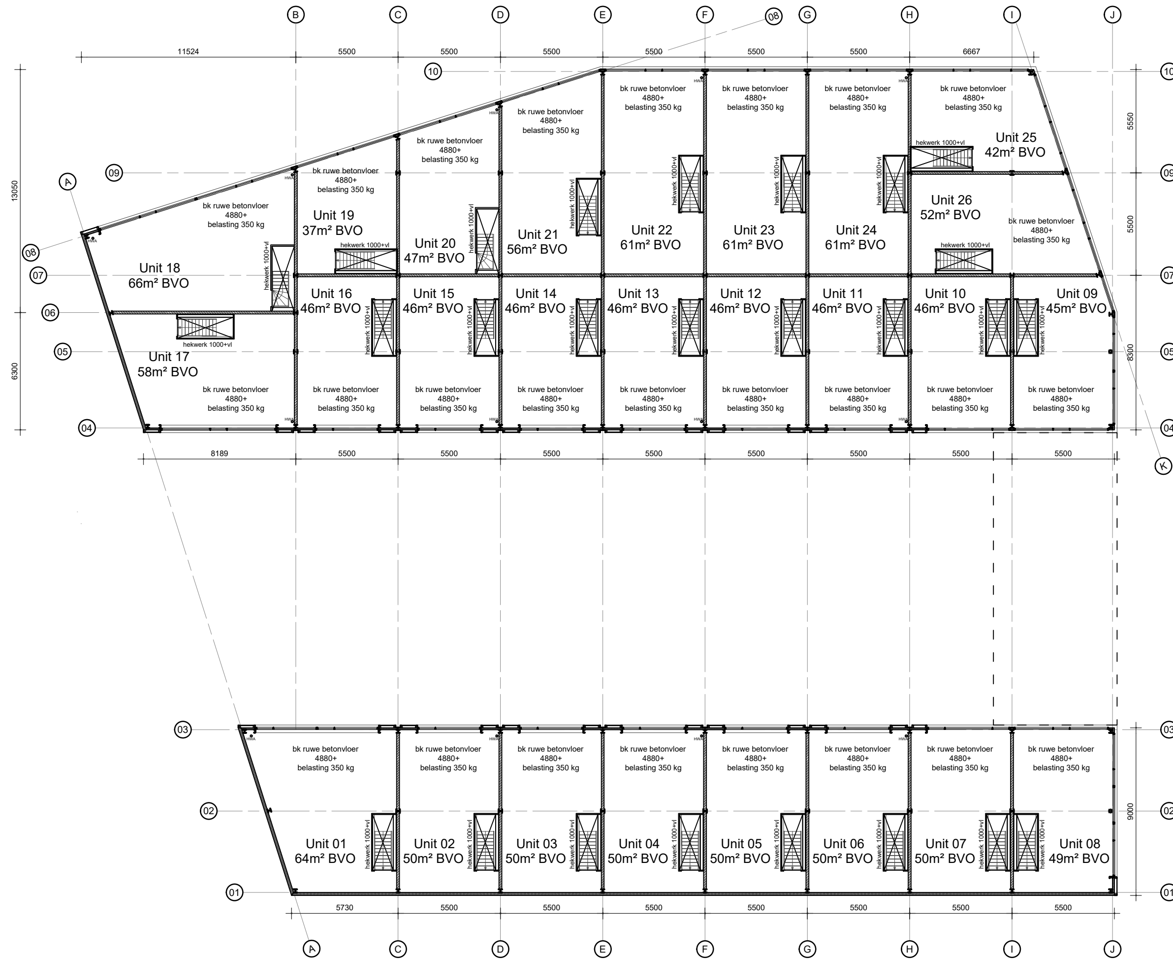
1e Verdieping 4880+
