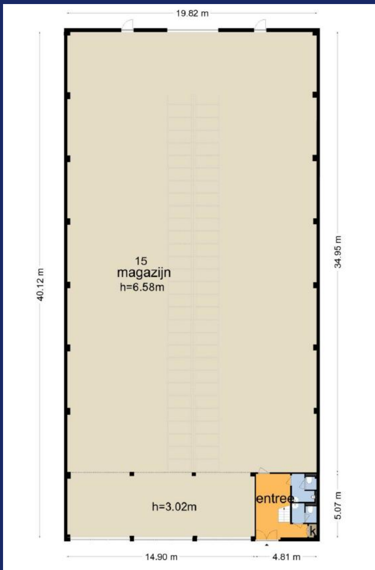
Begane grond
